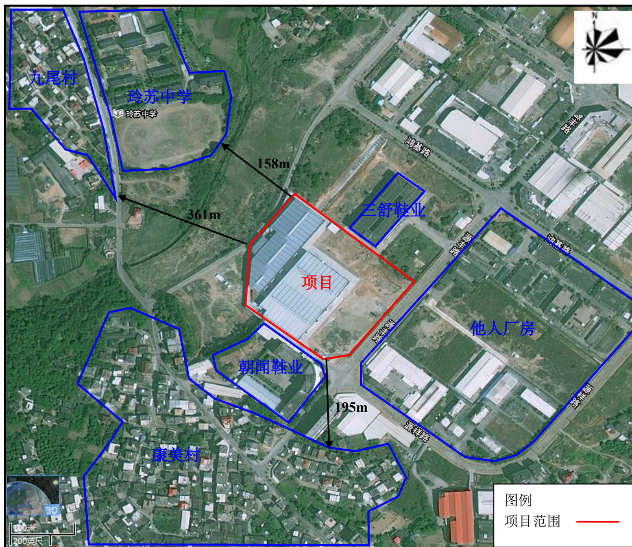
图 3-2 项目周边环境示意图
