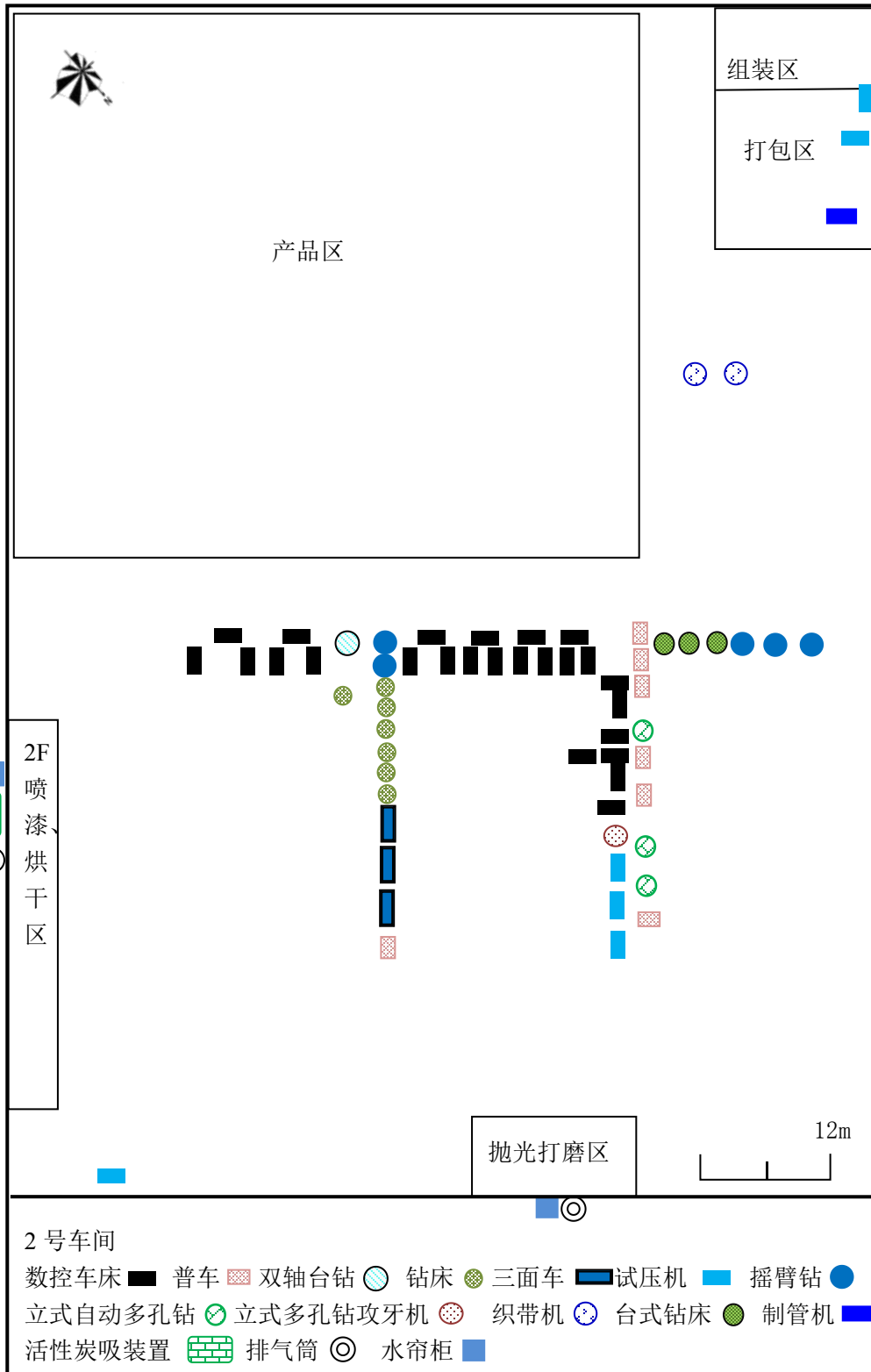
图 3-3 项目厂区 2 号车间平面布局图
